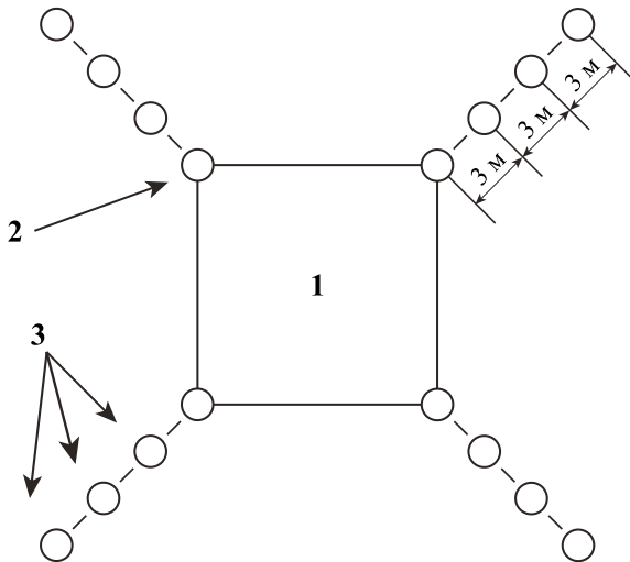
Рисунок. Обозначение рабочей площади вертолетной посадочной площадки без искусственного покрытия:
